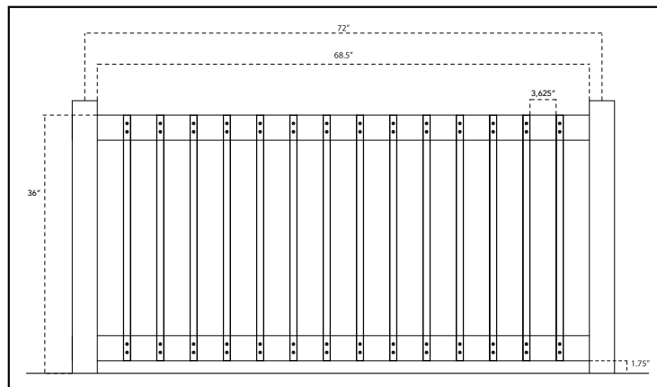
Railing Section / Section de rampe / Sección de barandilla
